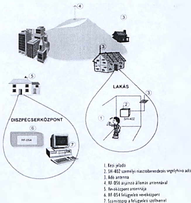
Jelzőrendszeres házi segélyhívó rendszerterve
