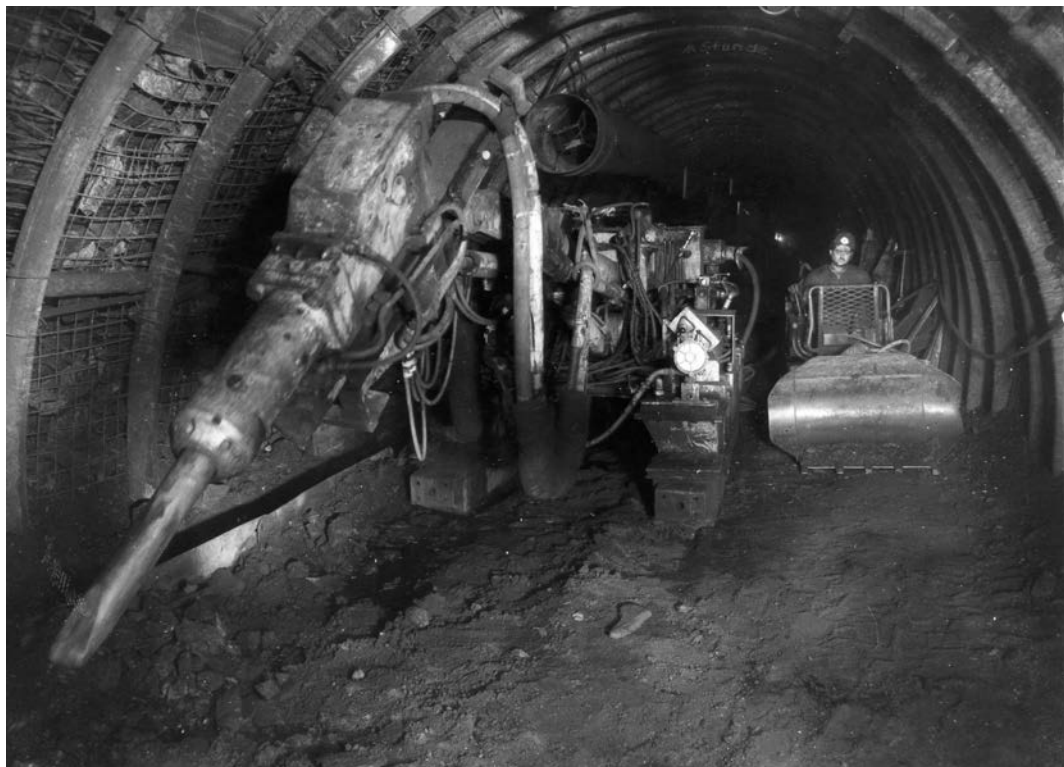
Az Impact Ripper vágathajtó gép, rakodókanál nélkül. Mellette egy Eimco 623-H rakodógép közlekedik.
