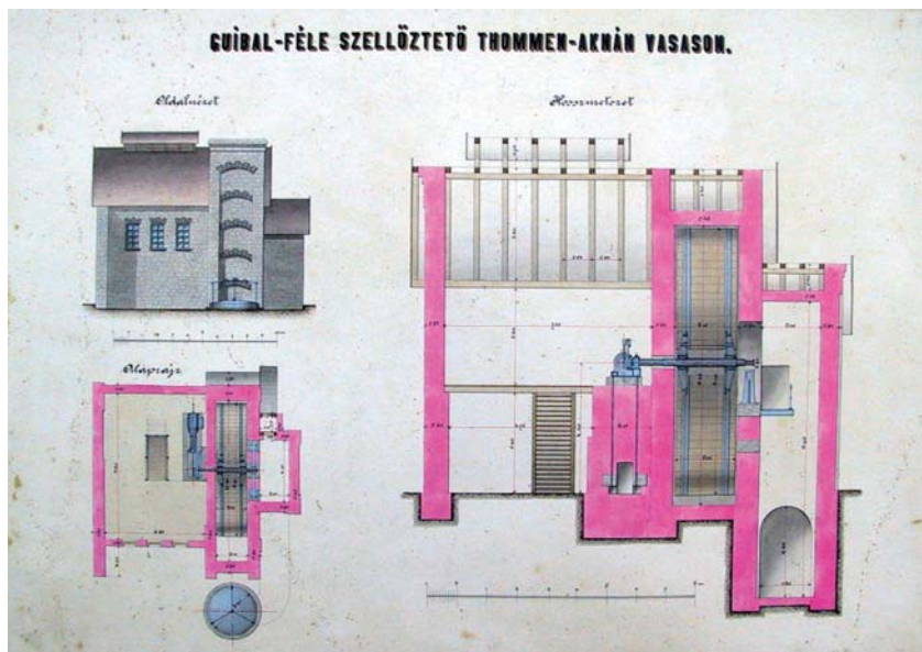
A Guibal szellőztető elhelyezése, metszetei
