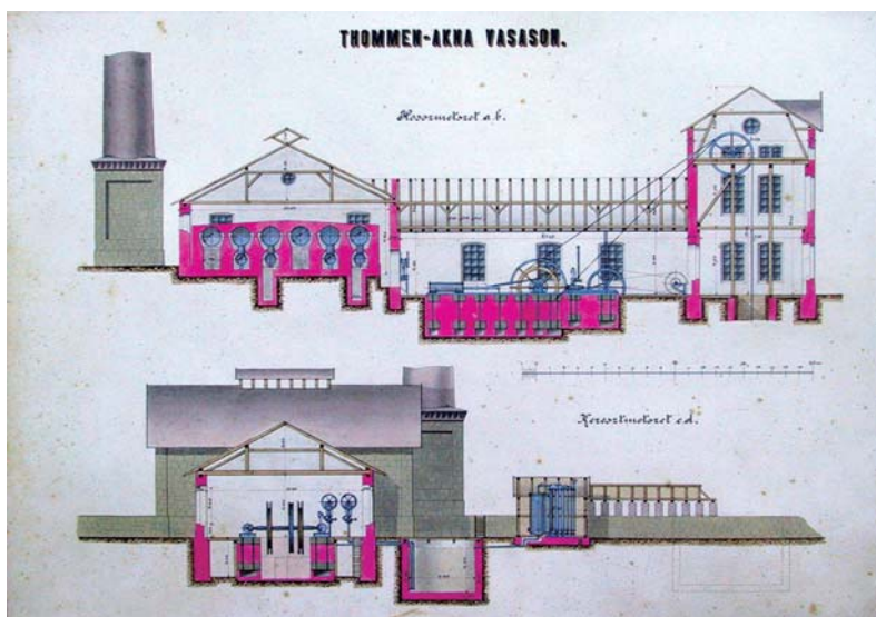
Thommen akna szállítógépházának metszetei
