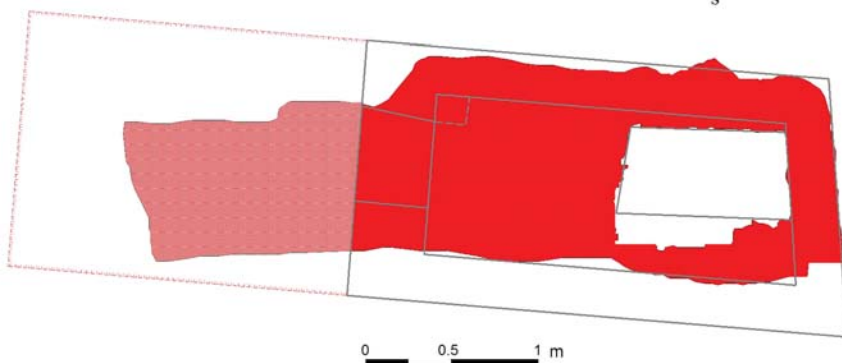
A sírípítmény alaprajza
