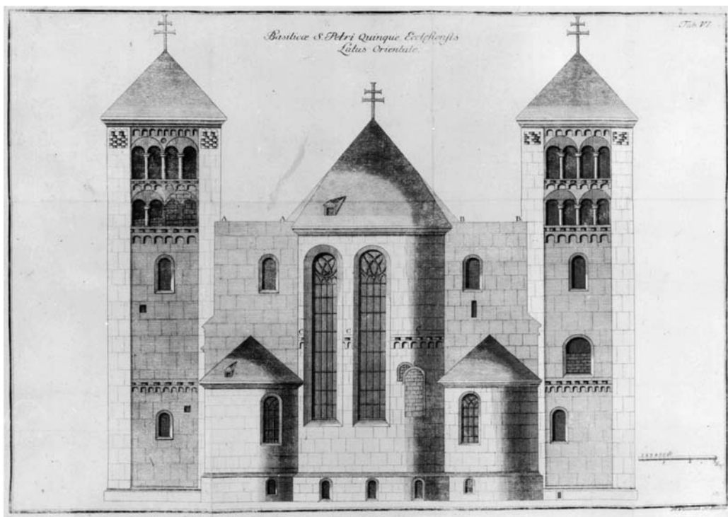
A székesegyház a 1804-ben, a székesegyház keleti homlokzata, Weinmann metszete
