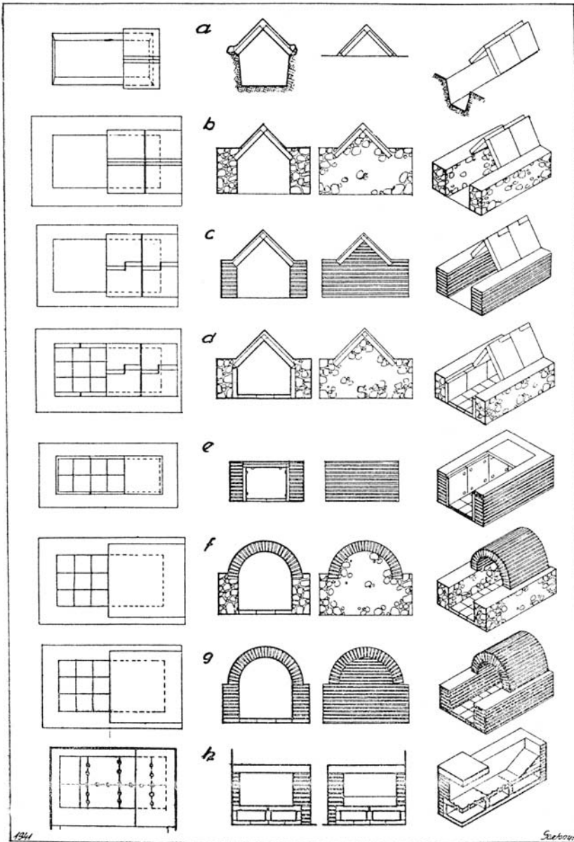
14. rajz. A pécsi római kori temető sírtípusai. a. földsír. b–d. falazott sírok nyeregvetővel, e. síkfödémrel, f, g. boltozattal, h. kettős fenékkal.
