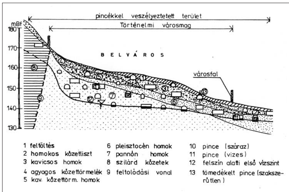
Mérmőkgeológiai szelvényvázlat alapincézett pécsi belvárosról.
