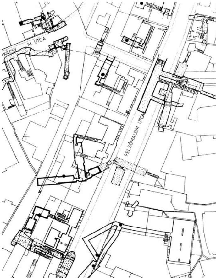
Közutak alá húzódó pincék Pécs belvárosában. A pontozott pincék már megszűntek.
