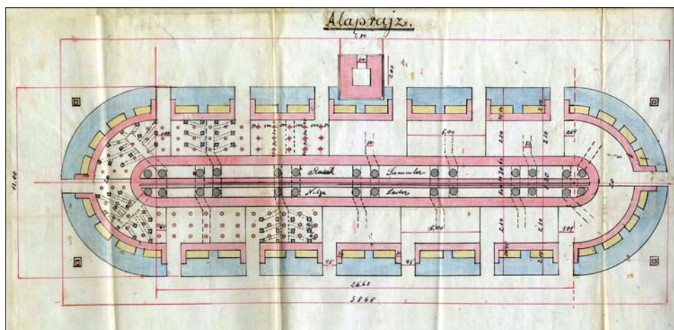
A mészégető körkemence terve, felülnézet
