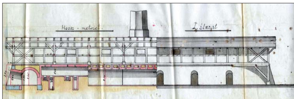
A mészégető körkemence terve, oldalnézet
