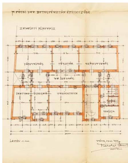
Károlyi Emil: A Pécsi Kerületi Munkásbiztosító Pénztár épülete homlokzata és emeleti alaprajza 1912.
