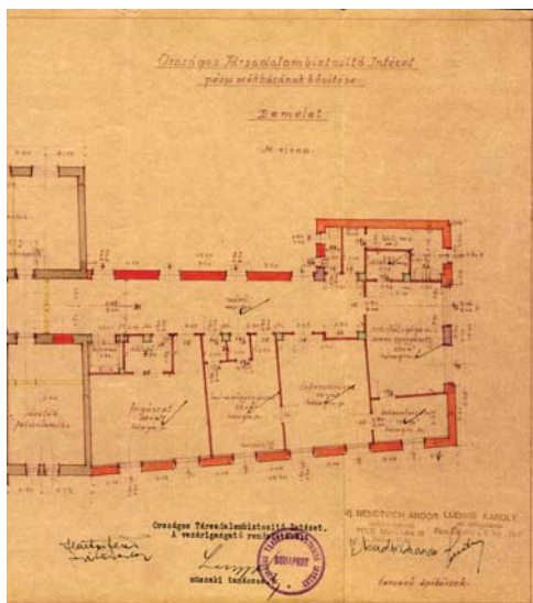
Az OTI Nendtvich Andor és Ludwig Károly tervezte bővítése 1938. Homlokzat és emeleti alaprajz
