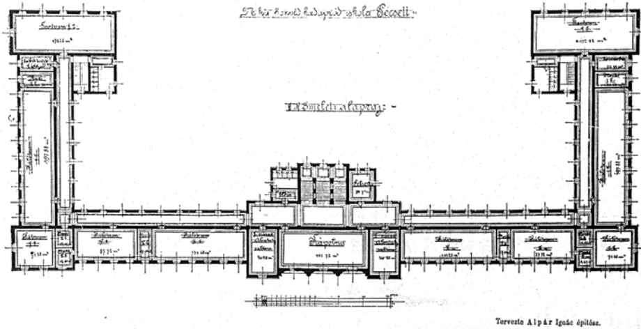
A Honvéd Hadapródiskola emeleti alaprajza.
