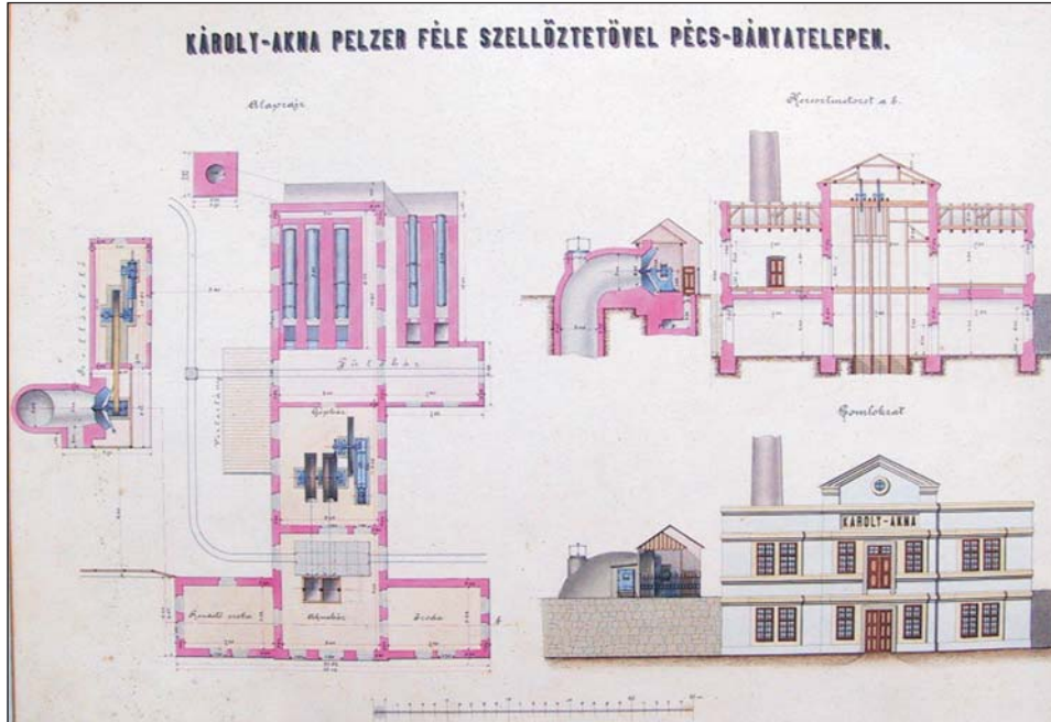
1. ábra: A Károly-aknai aknatorony-ház homlokzat-, metszet- és alaprajza a 19. sz. végén
