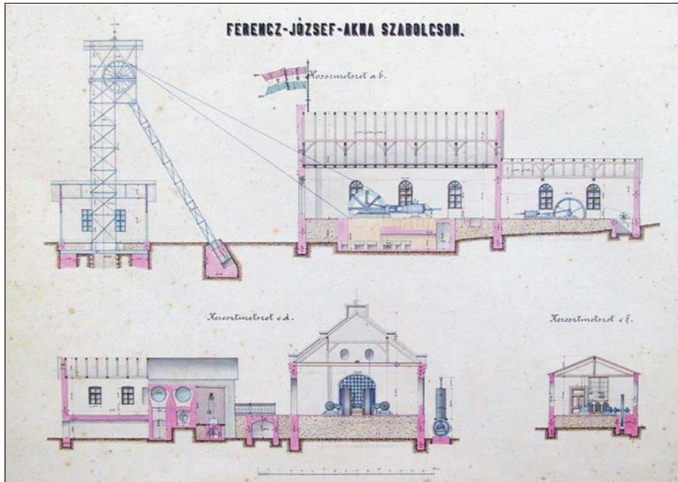
4. ábra: A szabolcsi Ferenc József-akna vasszerkezetű tornya és szállító gépháza a 19. sz. végén
