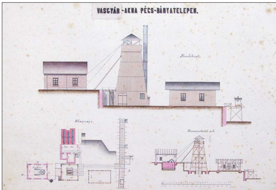
2. ábra: Vasgyár- (Zwang)-akna faszerkezetű aknatornyának és szállítógép-házának oldalnézet-, alap- és metszetrajza a 19. sz. végén
