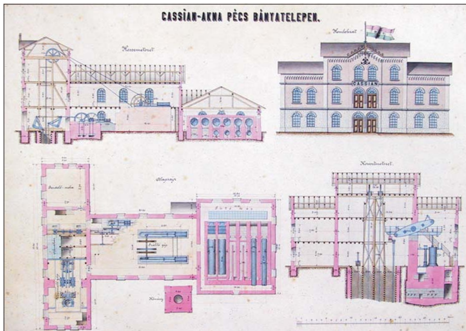
3. ábra: A Cassian-aknai aknatorony-ház homlokzat-, metszet- és alaprajza a 19. sz. végén
