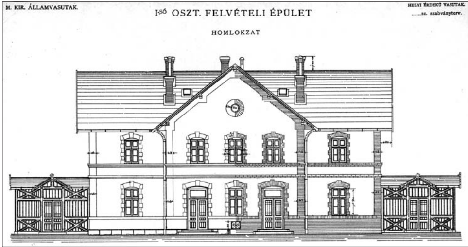
I. osztályú felvételi épület terve
