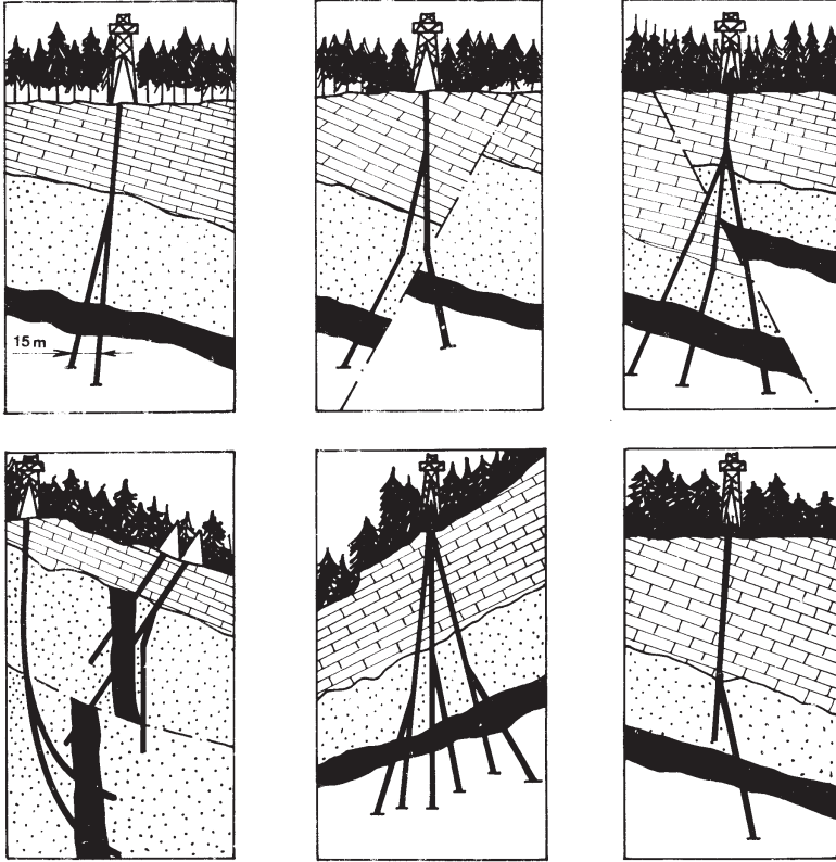
Irányított ferde fúrás
