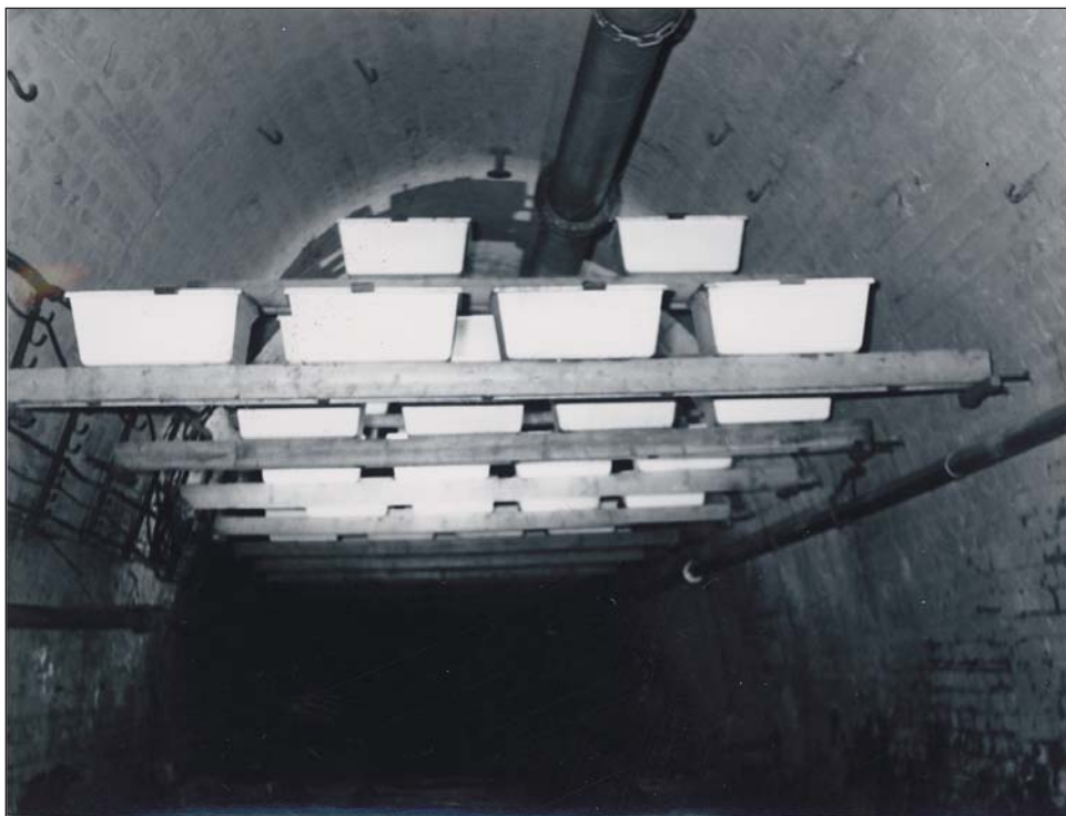
Robbanásfojtó vízzár egy bányavágatban.
