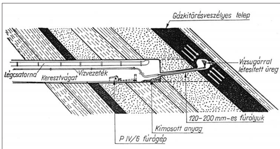
A gázkitörésveszély megszüntetése hidraulikus anyagkivétellel, telepharántolásnál
