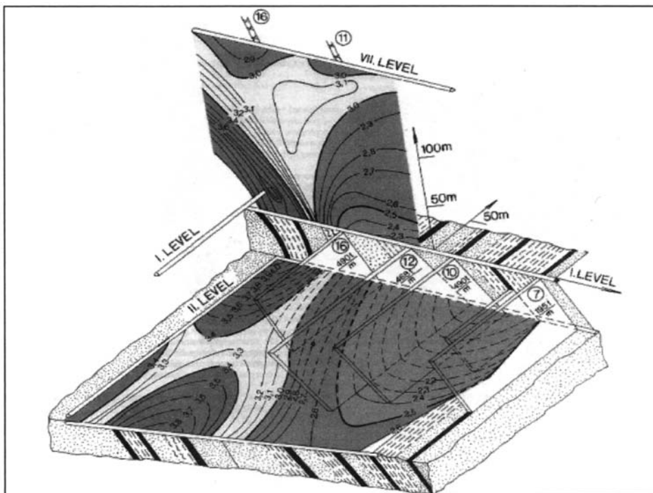
A fejtések környezetében lejátszódó kőzetfeszültség változások vizsgálata szeizmikus sebesség tomográfiával
