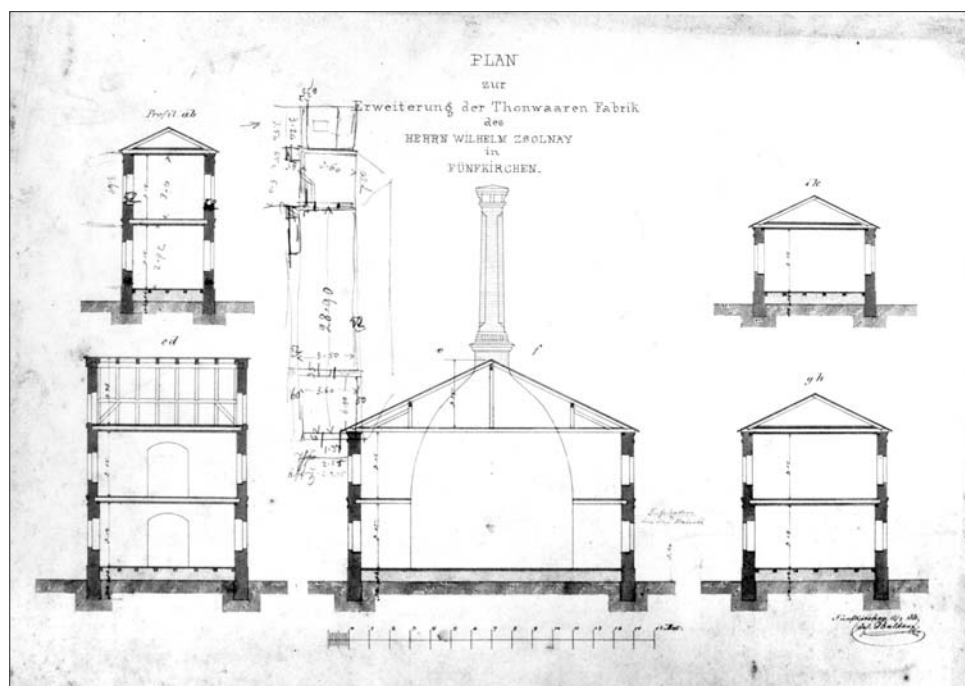
A Zsolnay gyári kemence- és műhelyépületek terve, 1881.
