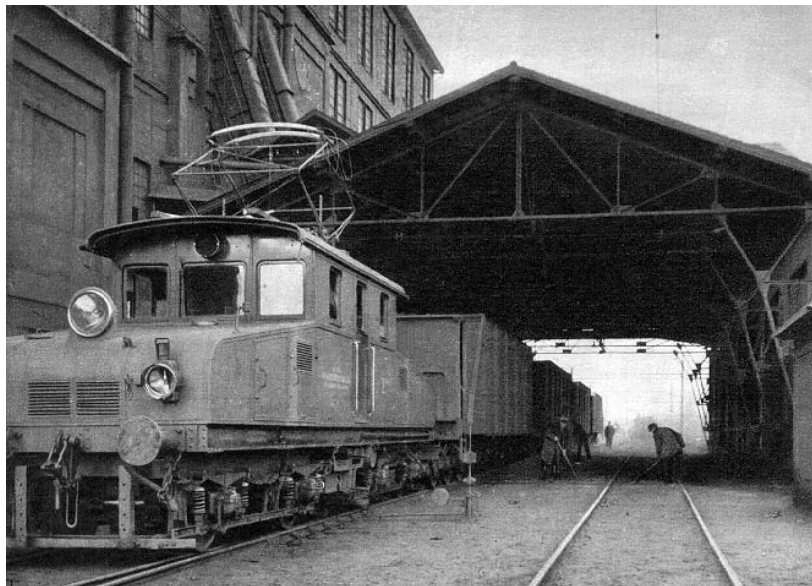
Szénfogadás az Előkészítőműnél
