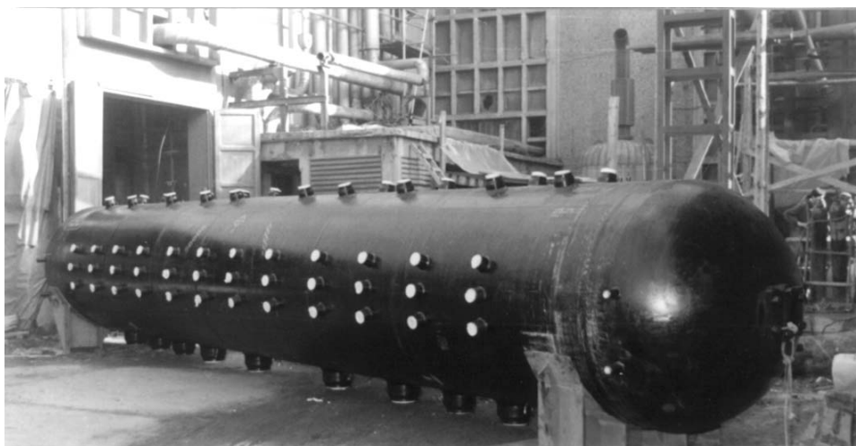
A 240 tonna/óra kapacitású kazándob beemelés előtt
