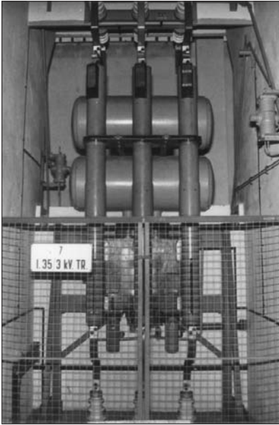
A 35 kilovoltos alállomás kapcsolója
