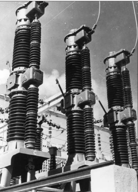
A 120 kilovoltos alállomás kapcsolója
