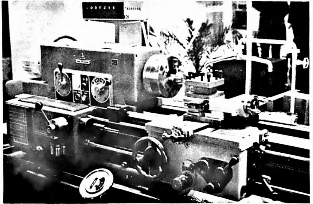
Egyelőre óhaj, de hamarosan valóságga válik, a képen látható esztergaped. A tavaszi BNV-n, a beruházási javak szakkvázisán láthattuk ezt a bolgár gyártmányú esztergapedot, amelyet vállalatunk meg is rendelt. Az új forgácsológép várhatóan még ebben az esztendőben megérkezik és a tmk-műhelyben lesz felállítva.
