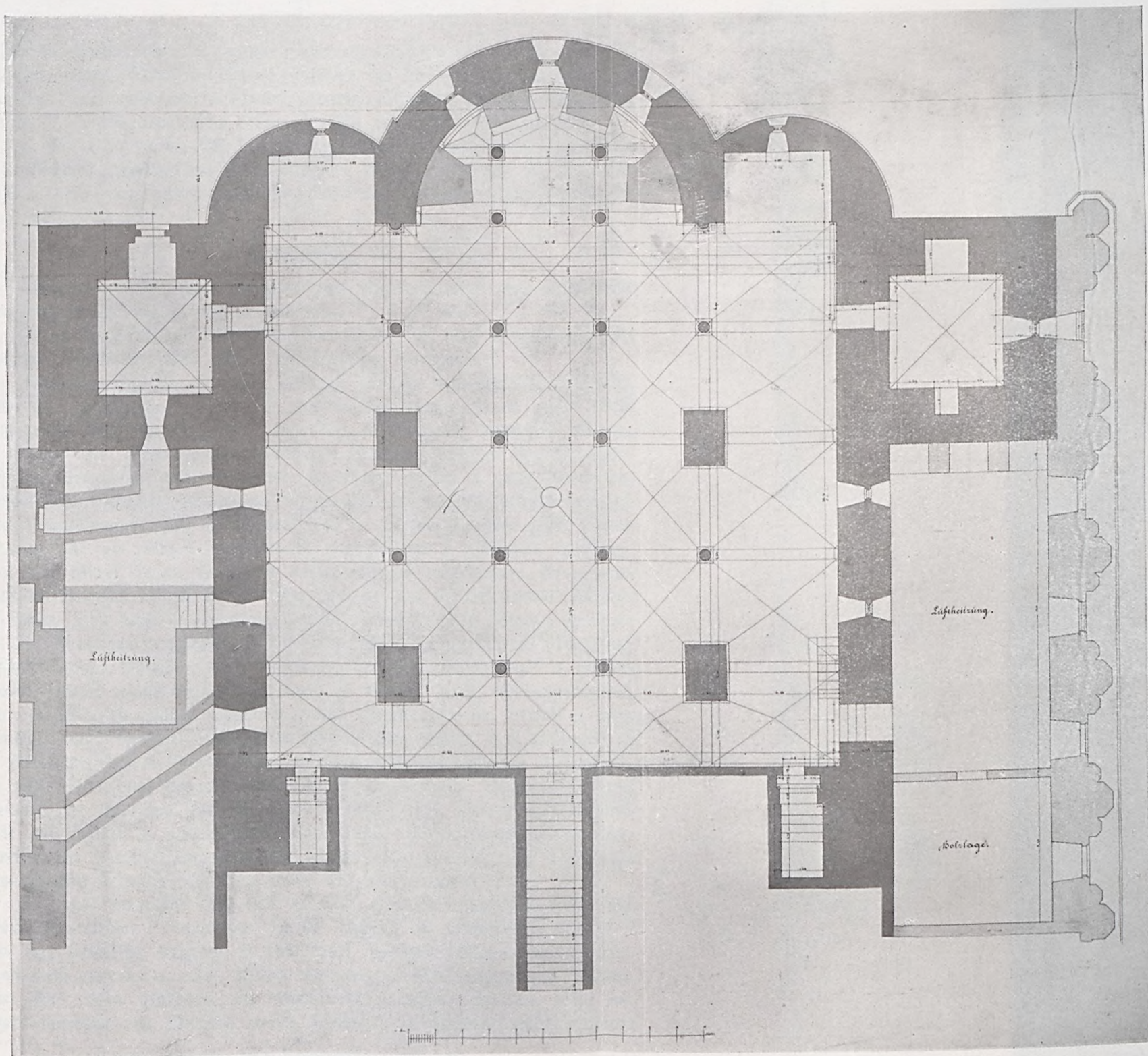
A pécsi székesegyház kryptájának alaprajza 1882 előtt.
