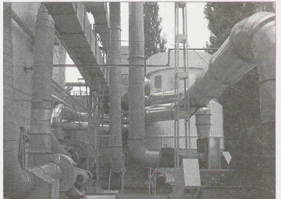
A mintegy 33 milliós beruházási költséggel telepített új porleválasztó rendszerben ciklofilter végzi a poros levegő szűrését. Fotó: Schindl
