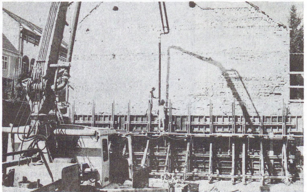
A Donauber Kft. végre megkezdte a belvárosi gödörben a betontámfal építését, miután sikerült a területet vízteleníteni. A munkálatok nagy intenzitással folynak.
