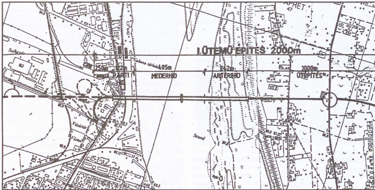
Mohácsi Dunahíd és kapcsolódó úthálózat az EXPO-híd utóhasznosításával
