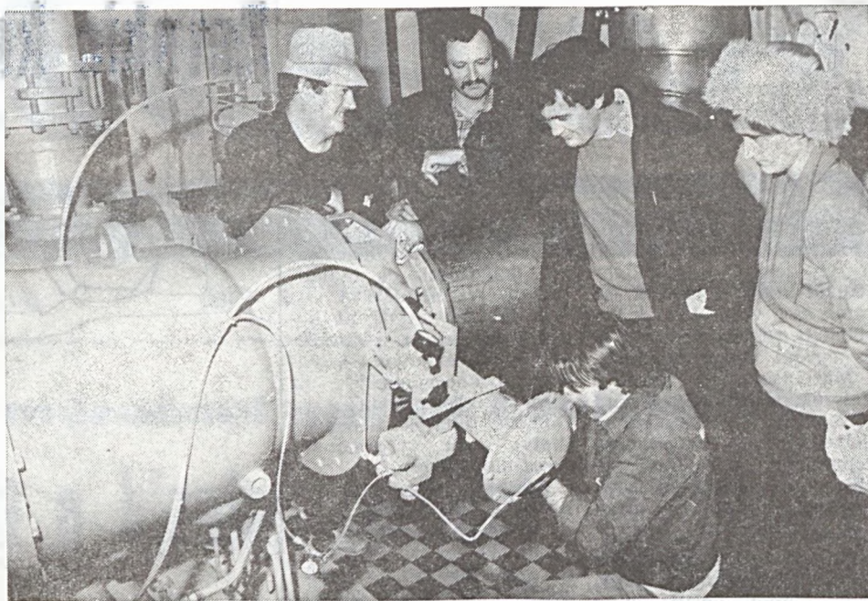
Az elmúlt év végén üzembe helyezték az EDÜ légsűrítő telepén egy INGERSOLL-RAND USA—olasz gyártmányú centrifugál légsűrítőt, mely vállalatunknál az első ilyen típusú gép. A dugattyús és csavaros légsűrítő ezzel szemben nagy előnye, hogy az EDÜ részére szükséges levegőnyomást olajmentes minőségben, nagyon jó fajlagos energiafelhasználással szolgáltatja. A géptől évente több mint 1 millió forint értékű energiamegtakarítás várható. Felvételünkön az üzemi technikusok és mérnökök gyűrűjében üzembe helyezési munkákat végez a szállító milánói Ingersoll-Rand cég képviselője. Keller Gábor
