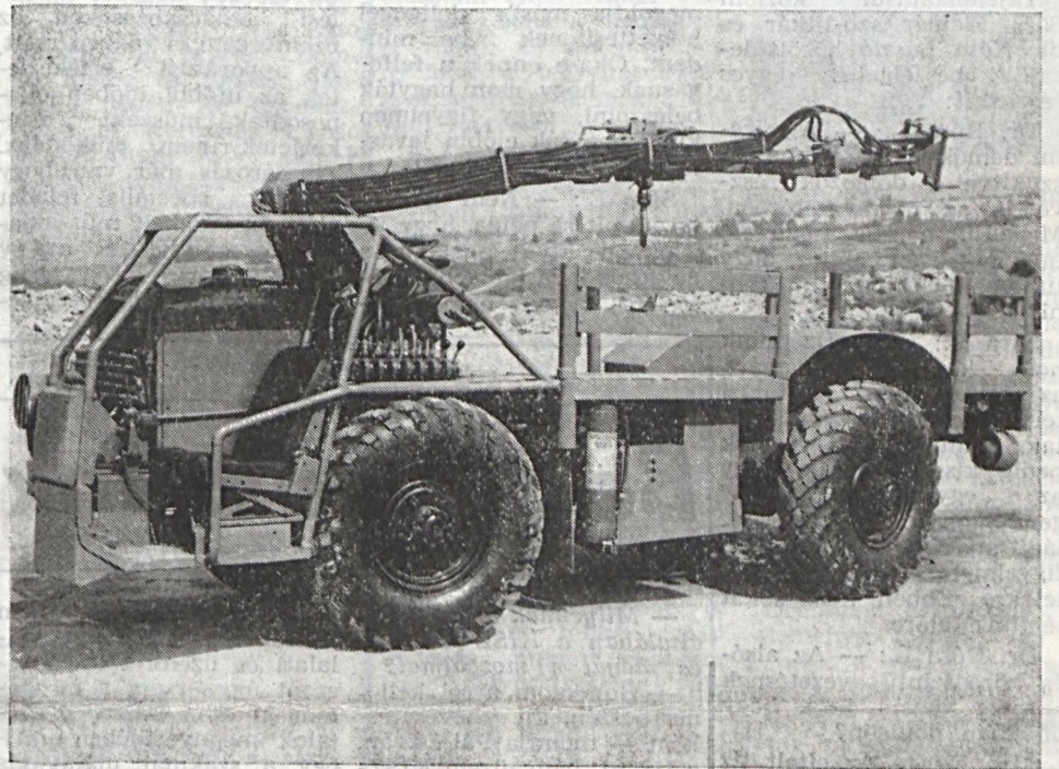
A dízel-üzemű kiszolgáló kocsit, amelyet vállalatunk Szolgáltató üzemében fejlesztettek ki, a jelenlévő szakemberek osztatlan elismerését nyerte el.
