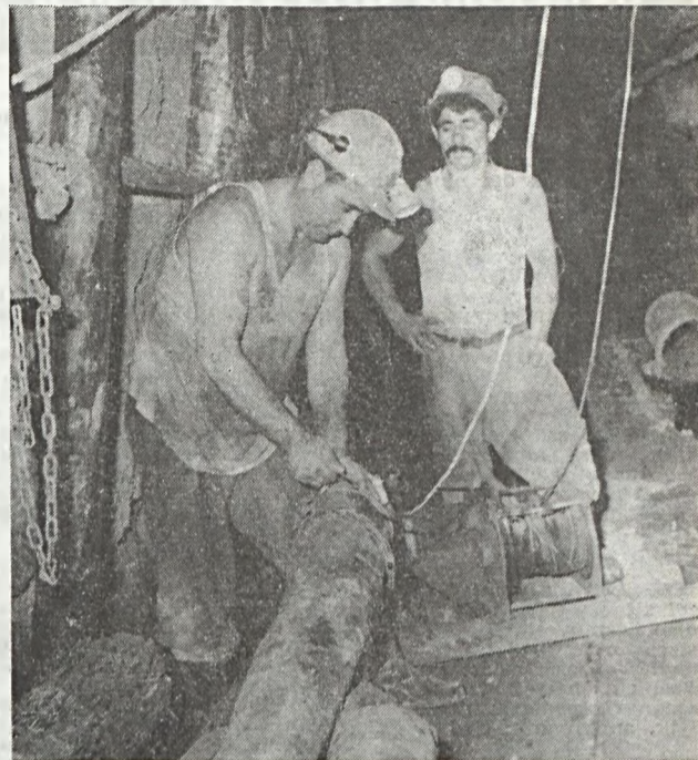
A feltöréshajtók. Balról jobbra Kotri Pál csapatvezető vájár, és Bertus Ferenc vájár a feltörés megbiztosításához szükséges keretfát húzzák vitlával. Bálint Jenő felvétele
