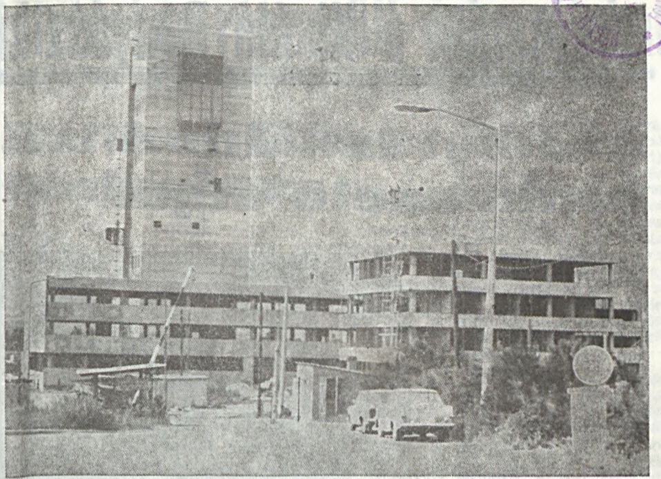
Megkezdődött az V. sz. bányauzem 56 méter magas aknatornyában a két darab KOEPE tárcsás aknaszállító gép szerelése. Az öltöző-fürdő és irodaépületek építését is rövidesen befejezik. Bálint Jenő felvétele
