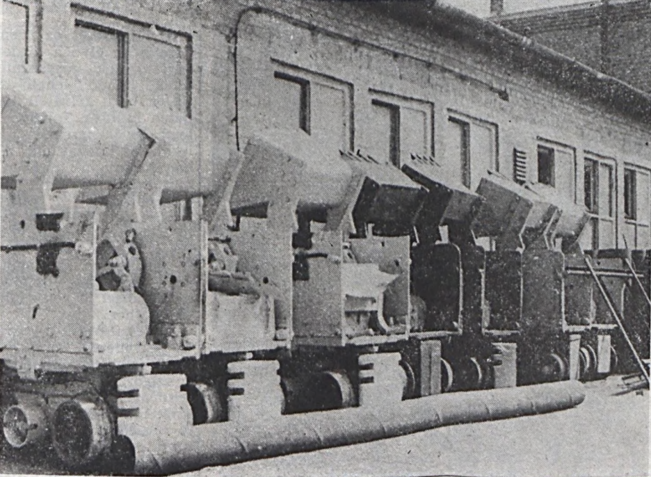
Felújított rakodógépek a Szolgáltató üzem udvarán
