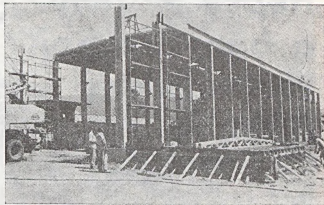
Új építési technológiával, úgynevezett „mezőpanel” szerkezettel készül a Szolgáltató üzemben az új bányagépjavító műhely. Réz Gyula felvétele
