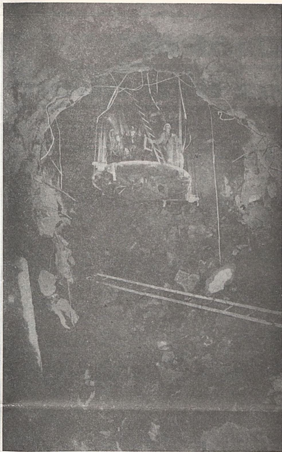
Július közepén fontos állomásához érkezett a IV. sz. bányüzemi új légakna építése. A Deák László vezette 71-es Váci Mihály ifjúsági szocialista brigád az Alimak bővítő padozattal elérte a tárorszintet. A fontos beruházási munka következő lépcsőjében innen folytatják az akna bővítést, előbb azonban az Alimakon elvégzik a szükséges nagyjavításokat. A bővítőpadozatot a tervek szerint szeptemberben helyezik ismét üzembe. A nagyjavítás ideje alatt a 71-es csapat hagyományos módon kezdi a visszabővítést a tárorszinten. Egy 25 méteres szakaszt így hajtának ki, ami azért szükséges, hogy a bővítőpadozat az első robbantásoknál ne sérüljön meg.
