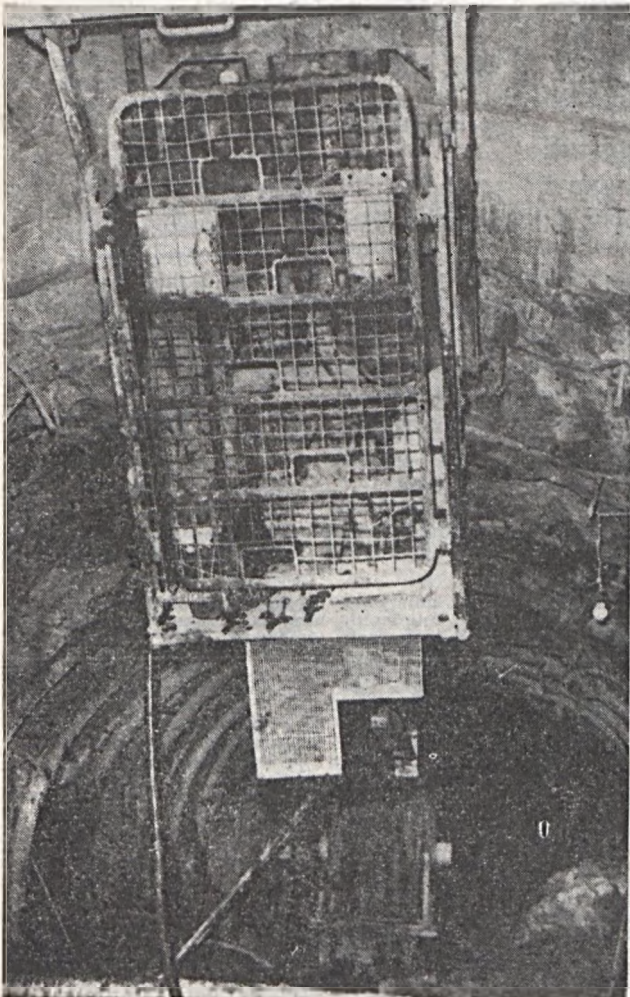
A III. sz. bányüzemben elkészült az a légfeltörés, amely a 10. és a 2. szintet köti össze. A 6,4 négyzetméteres szelvényű új légútvonalat a 69-es csapat hajtotta a déli akna közelében. A fontos beruházási munkához a képen látható KPV-1 B típusú feltöréshajtó padozatot használták.
