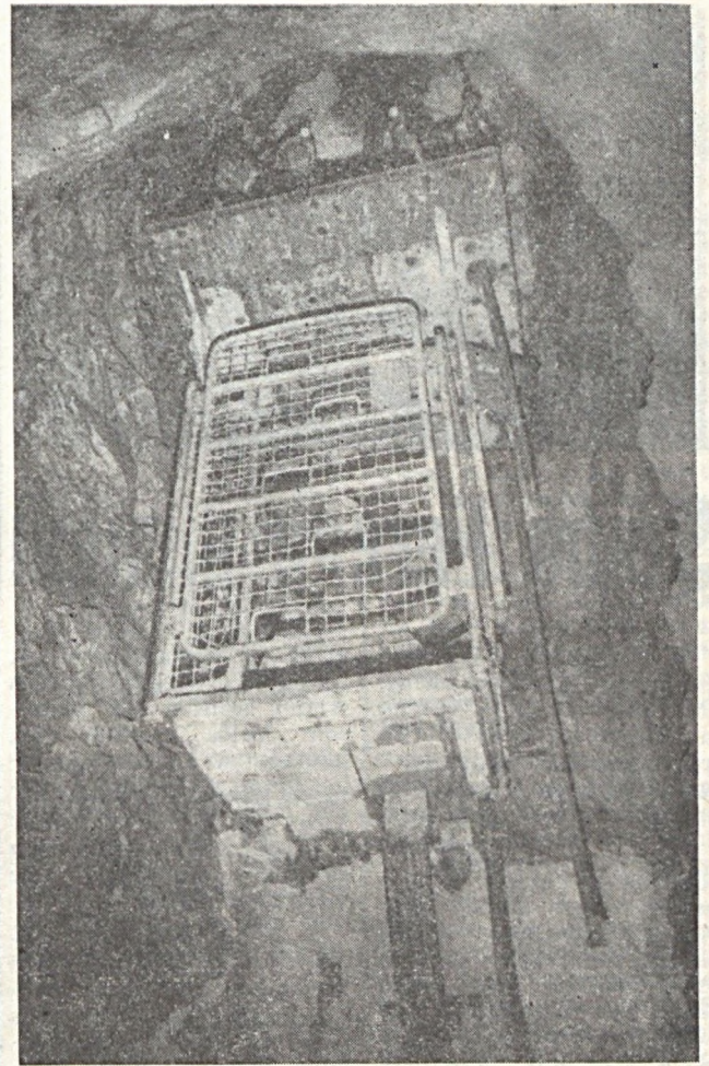
A KPV-1 B feltöréshajtó padozat. Csöndör László felvétele
