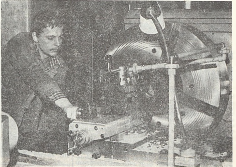
Az Ady Endre forgácsoló ifjúsági szocialista brigád egyik tagja, Magyar Sándor béléscső menetvágást végez. Egyed Imre felvétele
