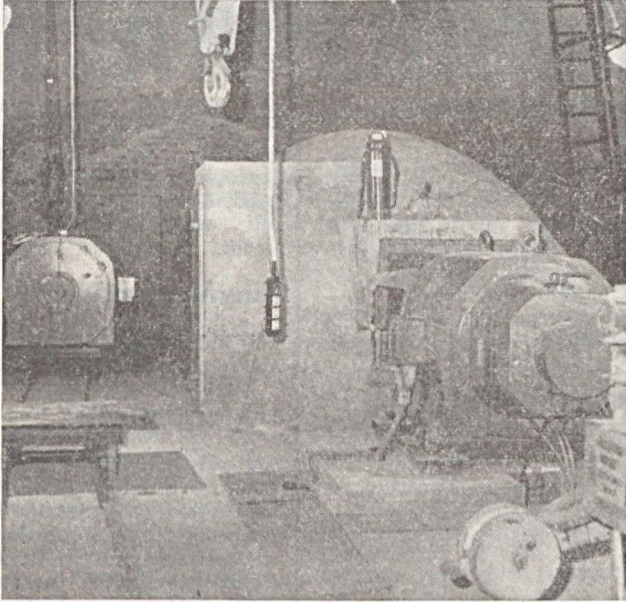
Működik a VOKD—2,4 típusú fűszellőtető gép a III. sz. bányában Szabó Győző felvétele
