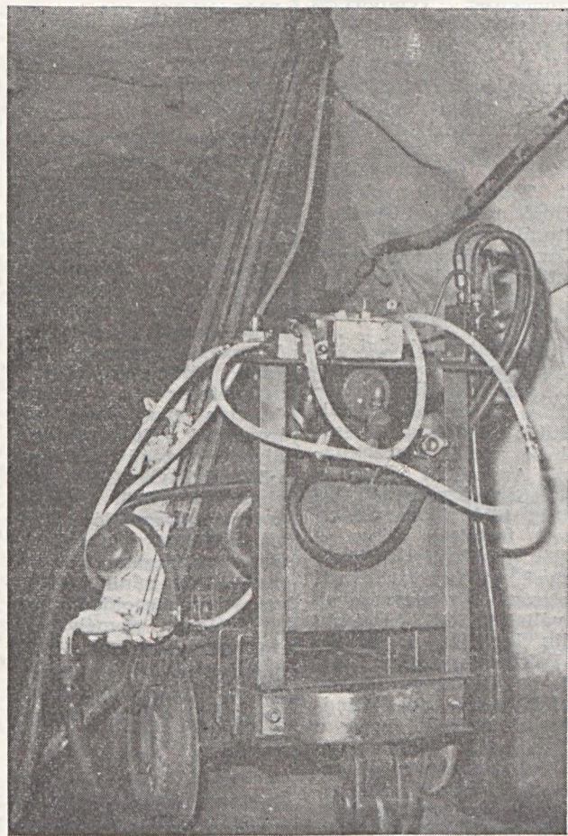
A könnyen manipulálható lafettával ellátott fúrókocsi szegecselőlyukat fúr
