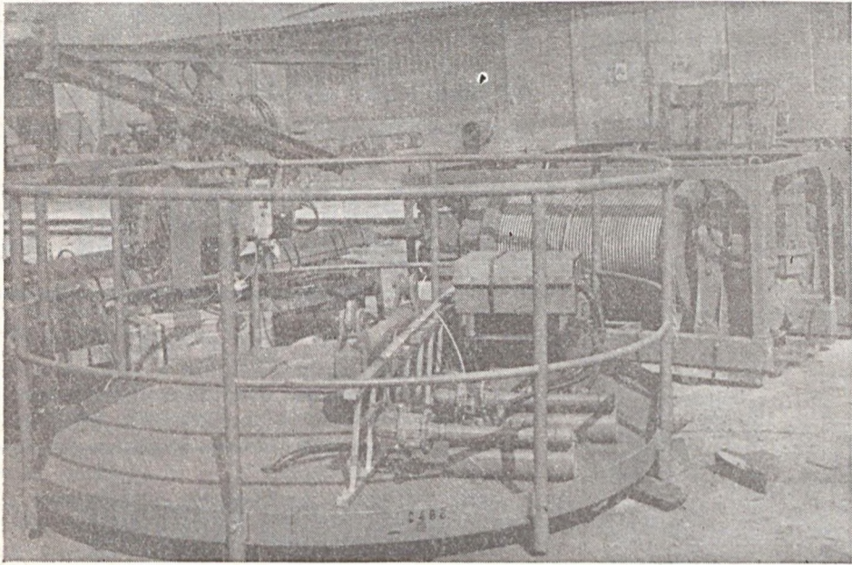
Az Alimak feltörésbővítő padozat az Anyag- és áruforgalmi főosztály udvarán Csöndör László felvétele
