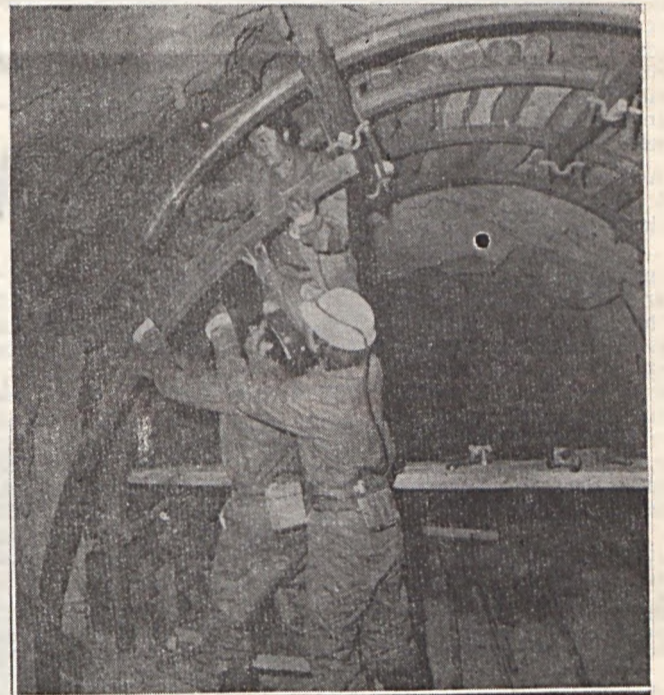
TH-ácsolat építés
