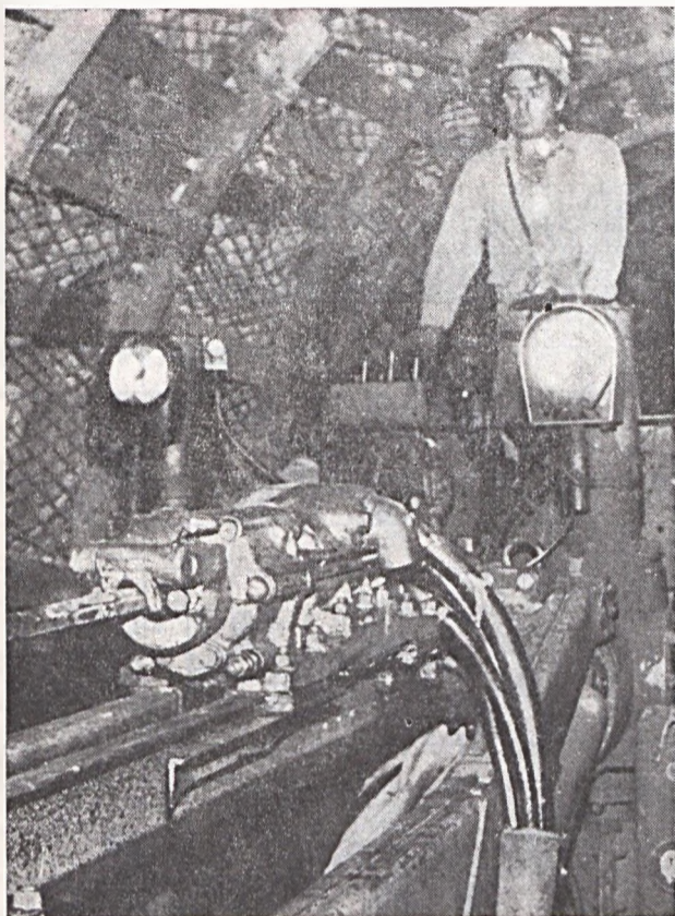
Horváth István csapatvezető a Minimatik fúrókocsin.
