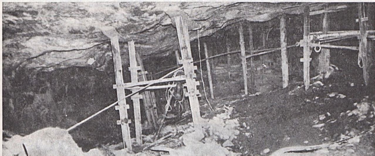
A fejtésben a fémtámok mint a szálfák meredeznek.
