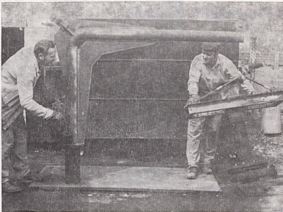
A dr. Münnich Ferenc szocialista brigád két tagja: Tólos Gábor (balról) és Molnár Lajos vertikális szivattyúkiemelő szerkezetet próbálnak ki az ÉDÜ III. üzemegységének lakatosműhelye előtt.
