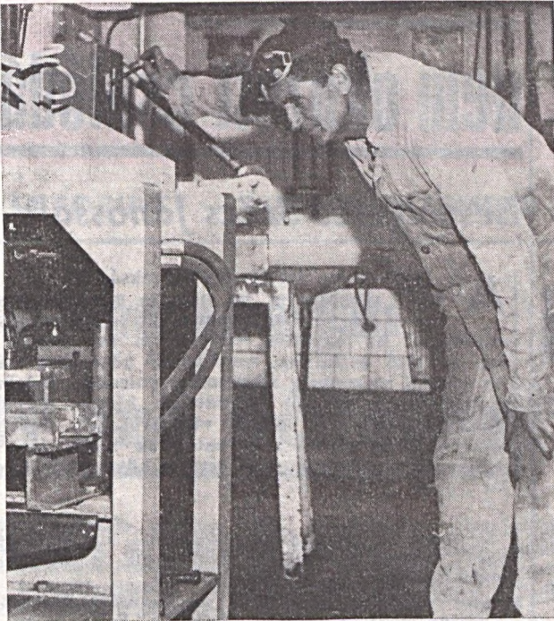
ScFDAY 16 típusú egytetemes hidraulikus daraboló géphez csatlakoztatható préselő és hajlító berendezést képiünkön Magyar János kezeli. Ez a gép sablonok alkalmazásával a mindennapi lakatos műhely munkáit nagymértékben könnyíti az ÉDÜ-ben. Kezelőjének újítótársa Balyi Ödön.
