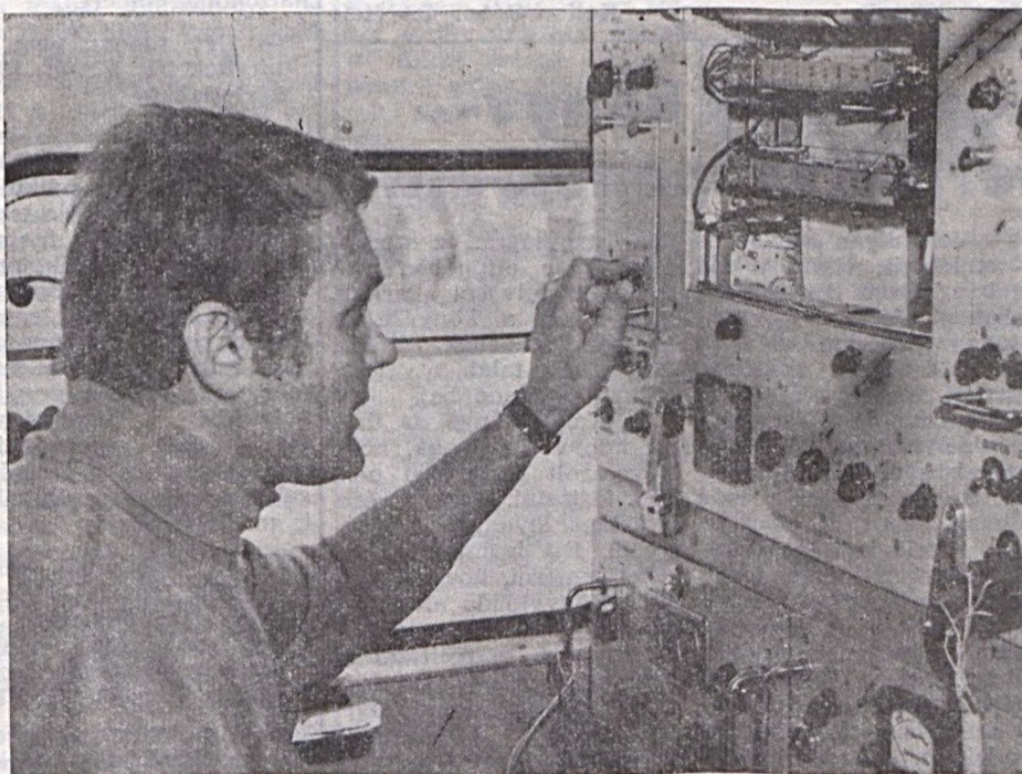
Faubel Antal észlelő a mélyfúrások geofizikai (karotázs) vizsgálatát végzi. Egyed Imre felvétele
