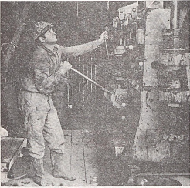
Simon László fűrómester rudazat kiépítést végez a Szigetvár 3-as vízkútjánál. Tér István felvétele
