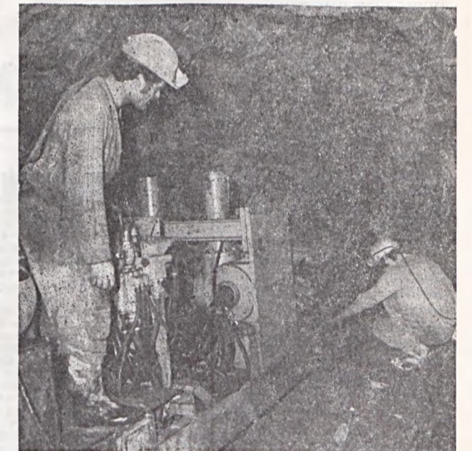
A IV. sz. bányázom Mezei Sándor karbantartó lakatos a Minirondó fúrókeci motortartó csapszegét szereli. Az ellenőrzést Sebestyén Imre csapatvezető végzi.
