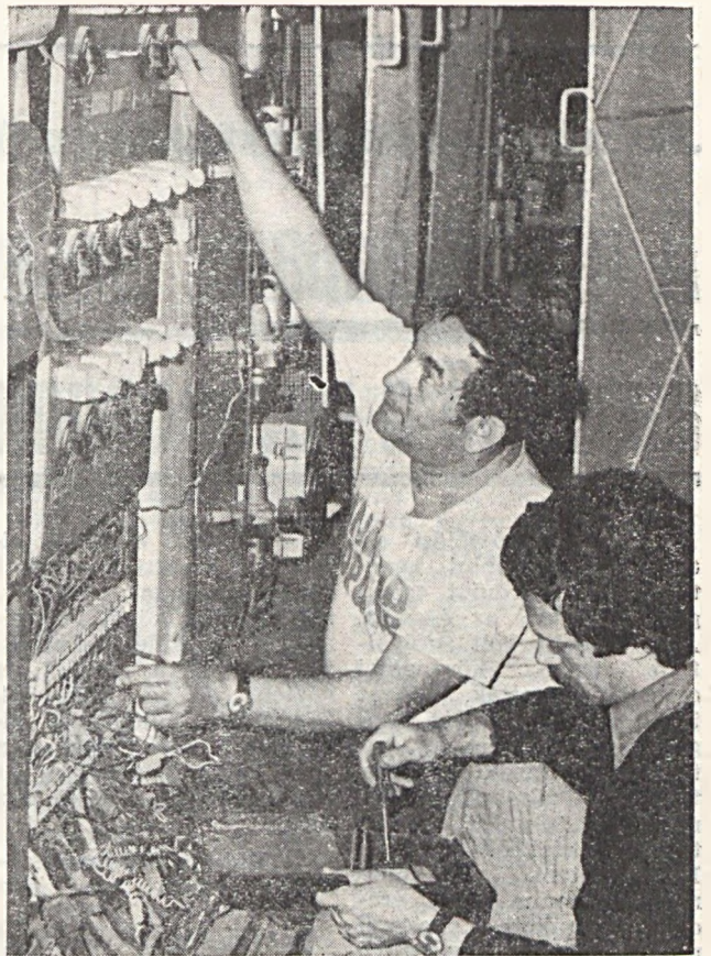
Az ÉDÜ üzemállása előtt a II. diszpécser helyiség kapcsoló tábláinak felújítását, illetve átkötéseit készítik elő Péter Géza és Berki Miklós műszerészek. Az Unio kéziműszer segít a kábelek behatárolásánál. Keller Gábor felvétele
