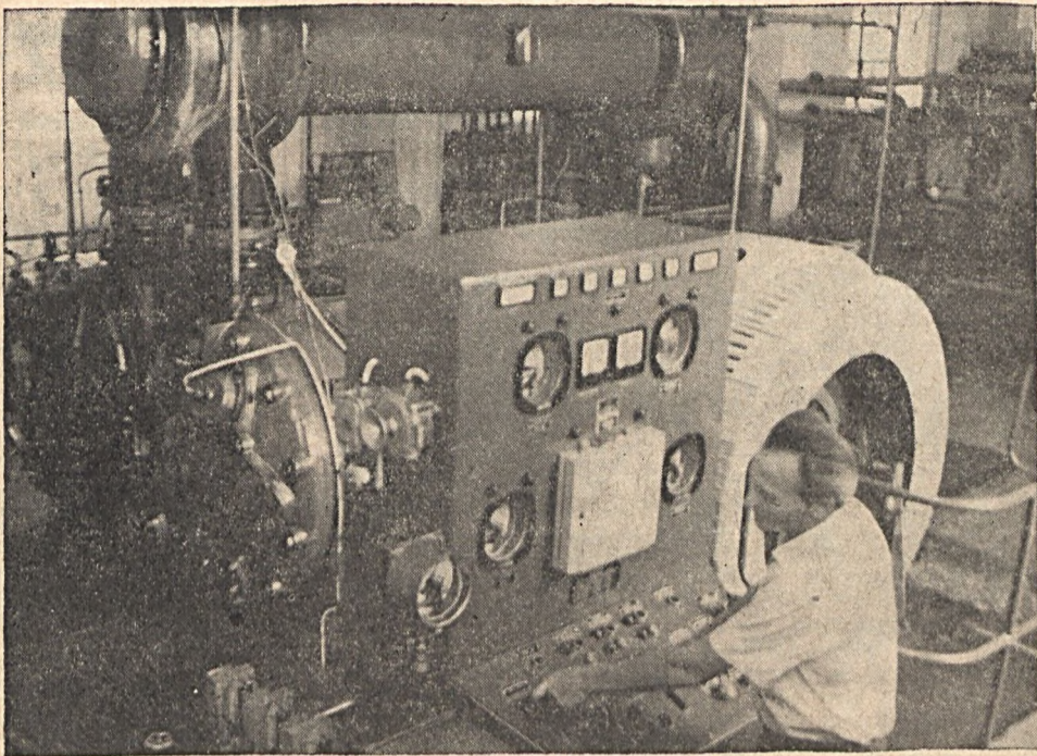
Ezek a nagyteljesítményű kompresszorok látják el levegővel a II. sz. bányászületet. A hatalmas csarnokban csak egy dolgozó teljesít szolgálatot. Képiükön a kapcsolópultnál Kiszner Kálmán kompresszorkezelő.
