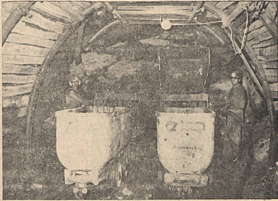
A II. sz. bányászület egyik duplaszelvényes TH biztosítású vágatában két rakodógéppel rakodik Káposztási János és Kisgyörgy István vágár, a 32-es szocialista brigád tagjai. Keller Gábor felvétele
