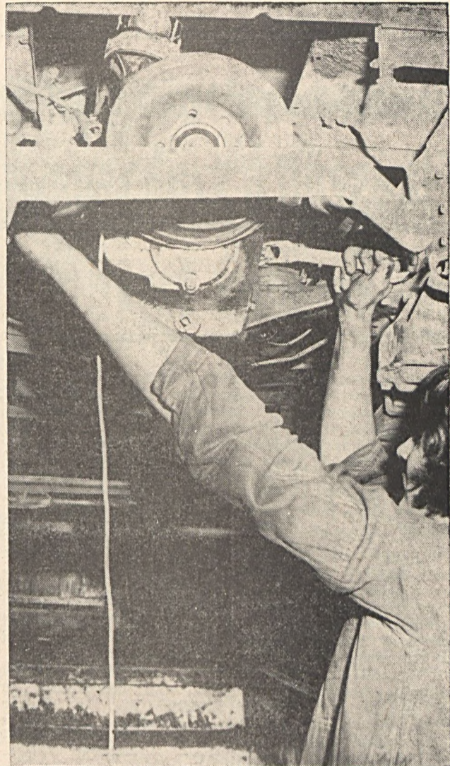
A Szolgáltató üzem gépkocsiszállítási üzemegysége végzi a II-es revíziót a vállalat gépkocsijain. Felvételünkön Bobány Sándor kuplung- és sebességváltót javít egy GAZ-53-as gépkocsin.
