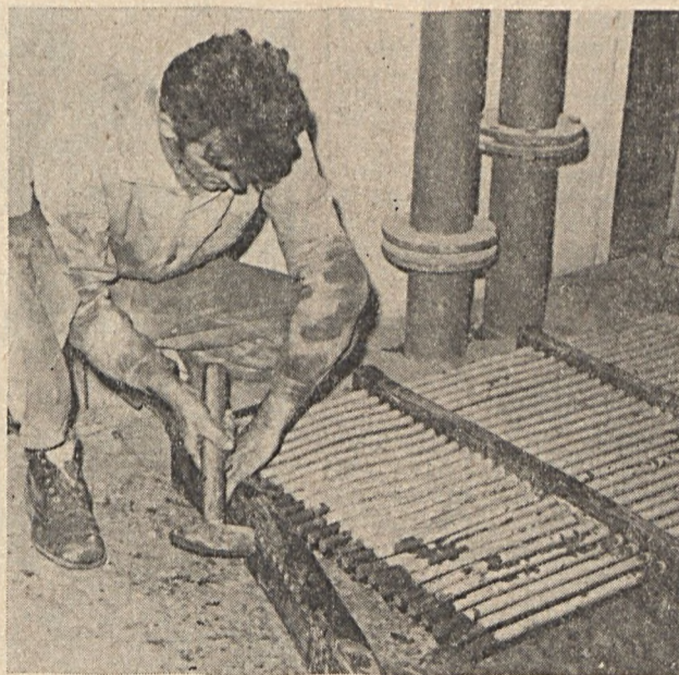
Egy minden tekintetben bevált újítás a zajcsökkentés, öntisztítás és élettartam növelés céljából, melyet még 1973-ban vezettek be az EDÜ-ben. A gumiba ágyazott acélhuzalos vibrációs ércosztályozó egység összeszerelését Sztranyák József lakatos végzi.
