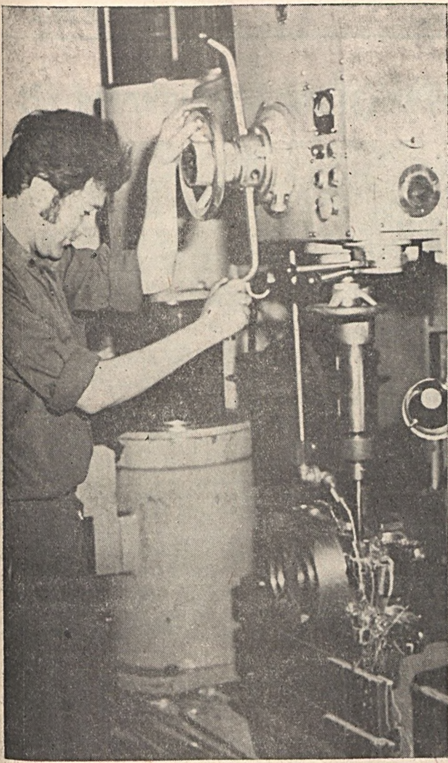
MHF-200-as közetfűró berendezés fordítókúpját készíti sugár-fűrógépen Teszari Árpád, a Szolgáltató Üzem dolgozója. Veress Tamás felvétele
