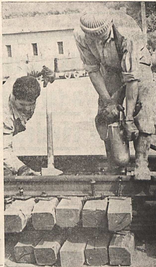
Fáy István és Haragovics János a bányabeli vasútépítéshez rakatokat (előre elkészített vasúti pályateszteket) készítettek elő. Veress Tamás felvétele
