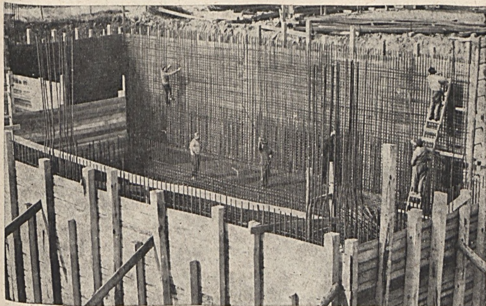
A Hídépítő Vállalat kivitelezésében egy korszerű zagykinyomató állomás épül az EDÜ területén Keller Gábor felvétele
