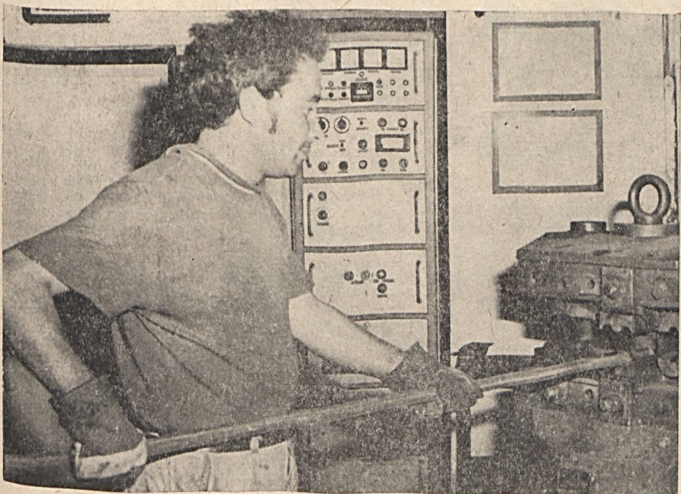
A fúrószár gallér zömítését végzi Kiss László a kovácsológépen.
