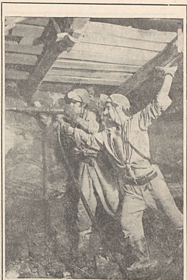
A IV. sz. bányászberuházásban Király Imre és Ruff János vajúrnak, az ideiglenes biztosítás „előtűzés” védelme alatt a meglazult kőzetdarabok lefeszégetését végzik fejtőkalapáccsal. Keller Gábor felvétele
