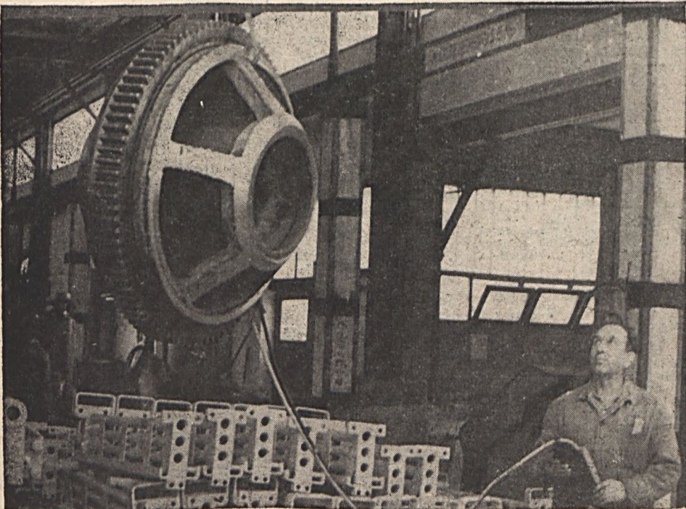
Egy tömedékelőgépfogaskerekét „lebegtetik” a IV. sz. bányüzem gépműhelyében.
