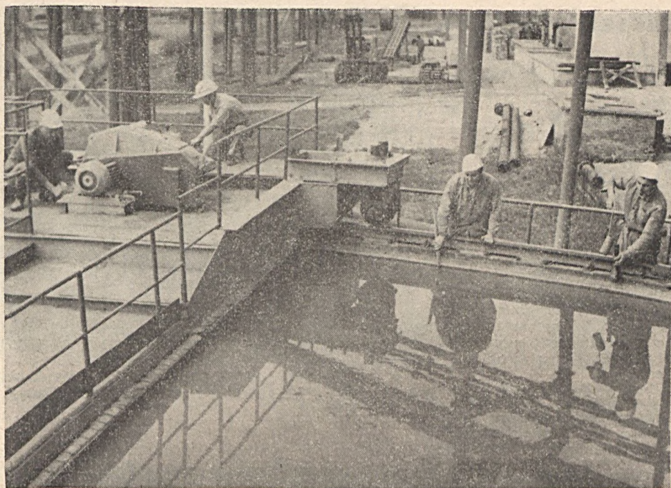
A Vállalat kiváló brigádja címet elnyert ÉDÜ Egyetértés szocialista brigádjának négy tagja: Hadobás Ferenc, Heller József, Molitor Ferenc és Aradi Ferenc a zagysűrítő dornál keverőszerelést, szint- és fajsúlymérést végeznek. Keller Gábor felvétele
