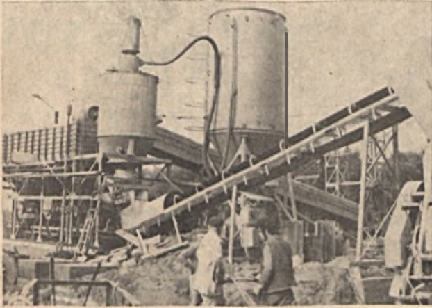
A szovjet 30 köbméteres teljesítményű betongyár megkezdte munkáját. Ezideig 42 méter akna betonozása készült el.
