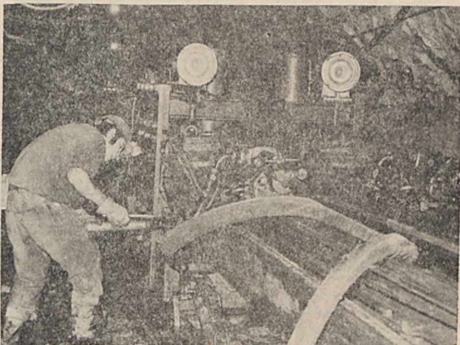
Miközben a csapat többi tagjai a kirobbantott kőzet csillékbe rakodását végzik a vágaton, a lakatos, a hátravontatott minirondó fűrókocsi karbantartásán dolgozik a III. sz. bányászaton. Keller Gábor felvétele
