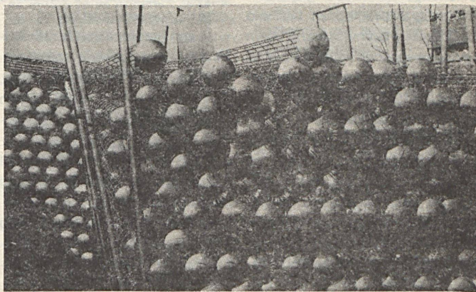
Folyik az új épület alapozása (fent). Beépítésre váró szűrőelemek (lent)
