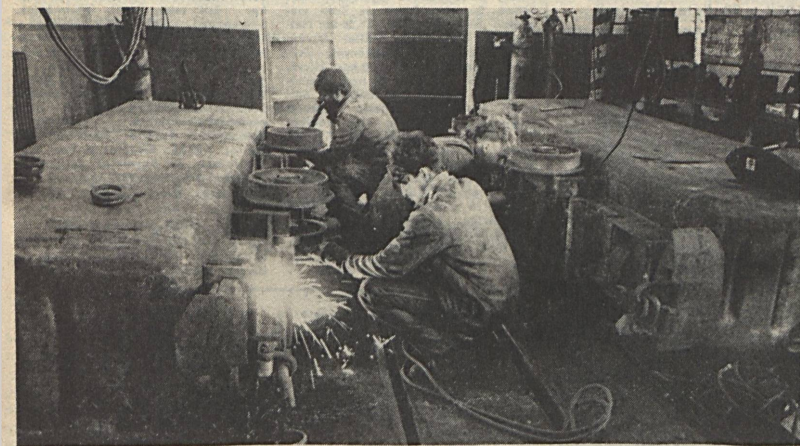
Az Anyagellátó Vállalat részére jelenleg már 8 főre csökkentett létszámban végez csillejavítást a magyarorszáki Egyetértés Mgtsz. Ez a kapacitás egységmértű csillét számítva napi 26 helyrehozatalát teszi lehetővé. Felvételünkön a tsz szakemberei kerékbilincs-hegesztés közben. Fotó: Tóth L.
