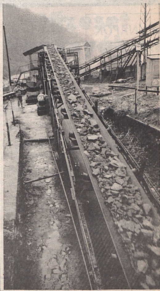
Dolgozik a meddőkihordó-szalag a Pannolit komlói kőbányájában Fotó: Tóth László
