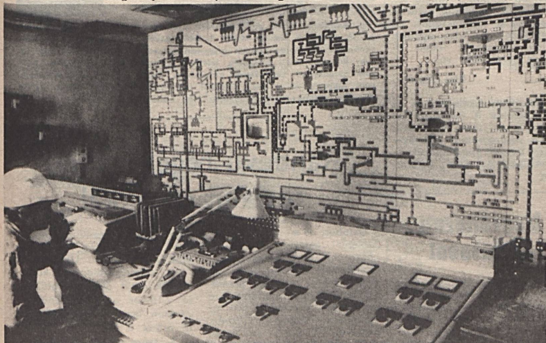
A Szénelőkészítő Üzemben korszerű irányítóközpont segítségével kísérik figyelemmel a munkahelyek szereteágazó tevékenységét.
