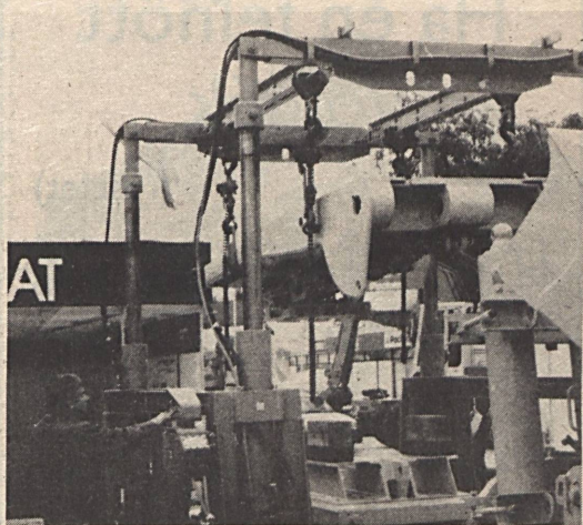
A Borsodi Szénbányák által kifejlesztett pajzsszerelő berendezéssel egy-egy egység összeállítása 4-5 óra alatt elvégezhető.
