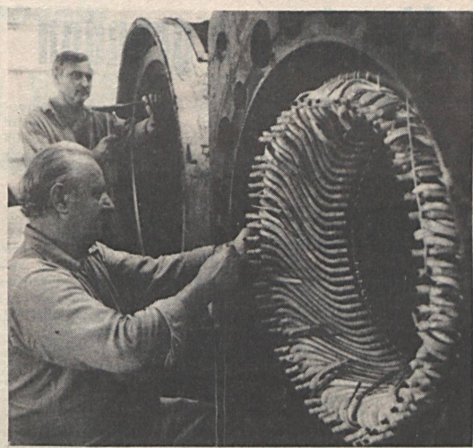
A Villamos Üzem szerelőműhelyében Bulsz Péter és Dunai Ferenc a Ward-leonárd szállítógép meghajtóegységének motorját javítja. Fotó: Kóródi Gábor
