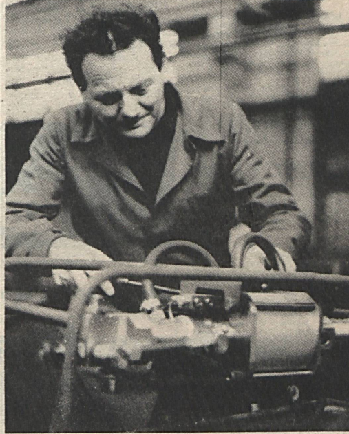
Hering János és Lang Ádám, a Központi Gépipari Műszaki Vezetői Tanács fejlesztették Varga Lajos és Krasz Imre már elfogadott újítását, a habziváltót. A módosítás lényege, hogy a habképző anyagok arányát tetszés szerint lehet beállítani. Konstrukciójában is módosult, mert differenciálüzeművé vált a hab anyaga. Fotó: Kórádi
