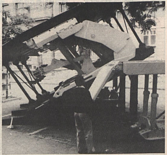
A Mecsek—Veszprém—Dowty—Dőlésmenti 120-as fejteszítősítő-berendezés a Pécsi Ipari Vásáron
