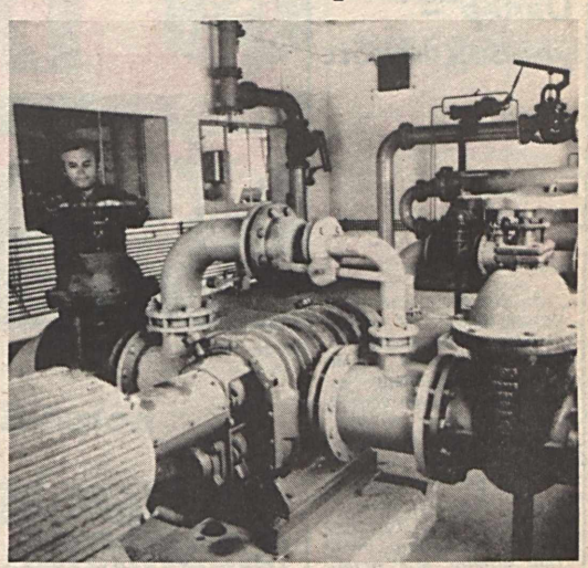
Vasason a gázlecsapolót ismét üzembe állítják. Közel 5 évig nem működött, mert a fejtések nem igényelték. Most, hogy az 5/A. szinti fejtés beindult ismét szükség lesz a gázlecsapoló be- vezetésére. A Mecseki Szénbányák Villamos Üzeme új vezérlő- pultot készített, a vasasok pedig a gázlecsapolásra új telepe- ket közel 100 méter hosszú furatokkal látta el. Havonta közel 90 ezer köbméter gázt szeretnének a telepből kihozni. Tervek is készültek az így nyert gáz további hasznosítására.
