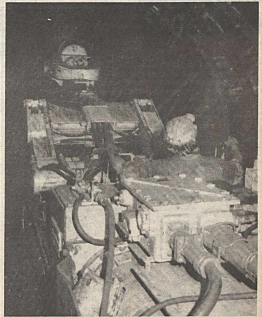
Reménykeltőek az első tapasztalatok Zobák-bányán a Webster 3000 CL vágathajtó gépről. Nemesi Árpád felvétele a bányában működés közben örökítette meg a berendezést.
